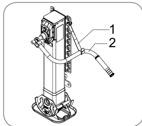
Abb. 6 - Kurbelfunktion
