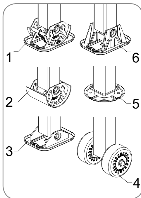
Abb. 5 - Zubehörteile SAF Hercules
