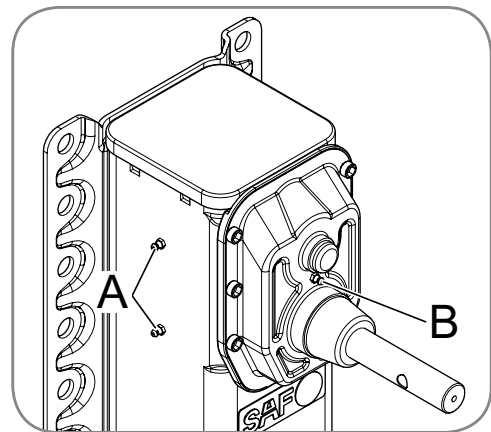
Abb. 8 - Stützvorrichtung abschmieren
