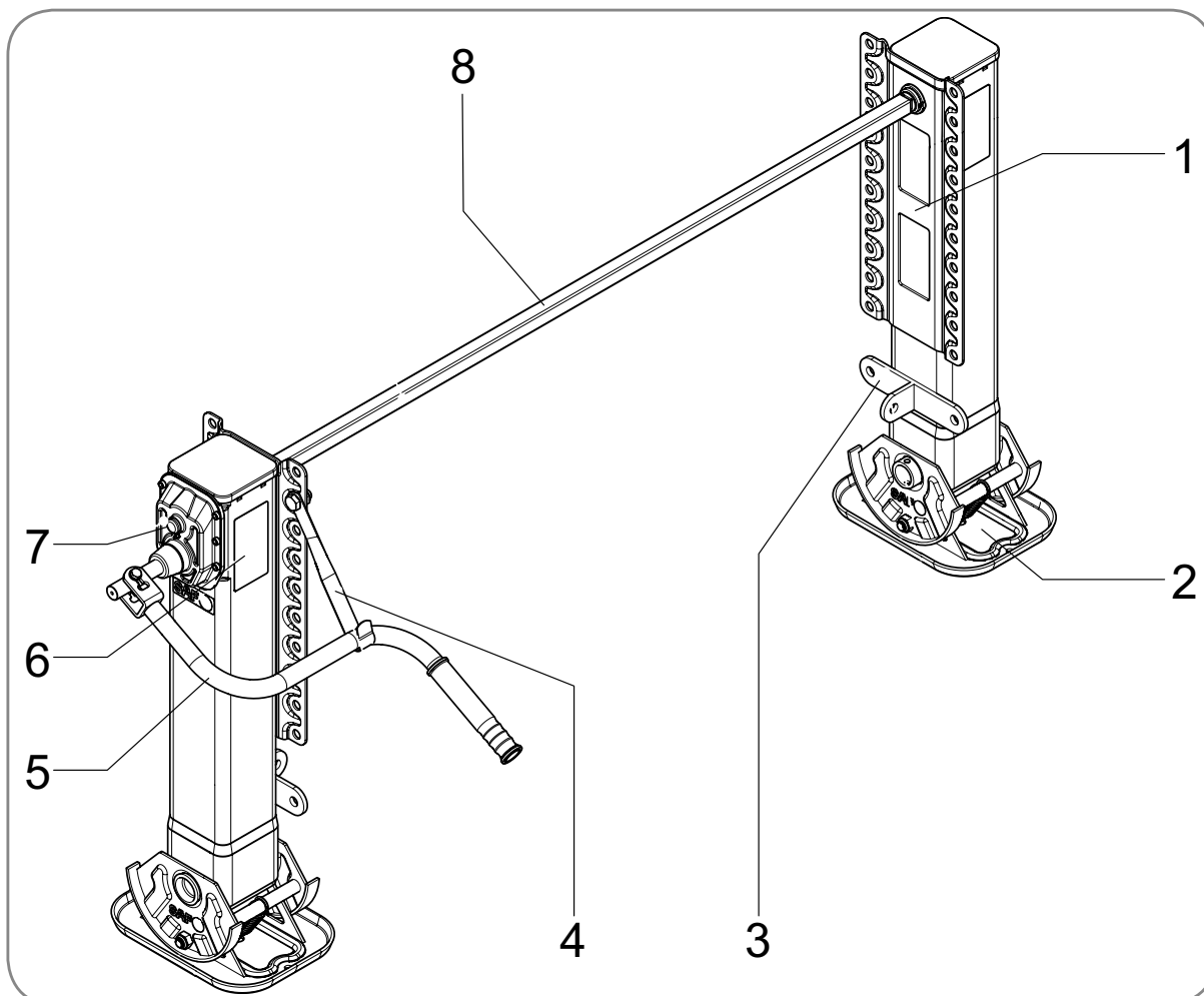
Abb. 4 - Bauteilübersicht SAF Stützvorrichtungen
