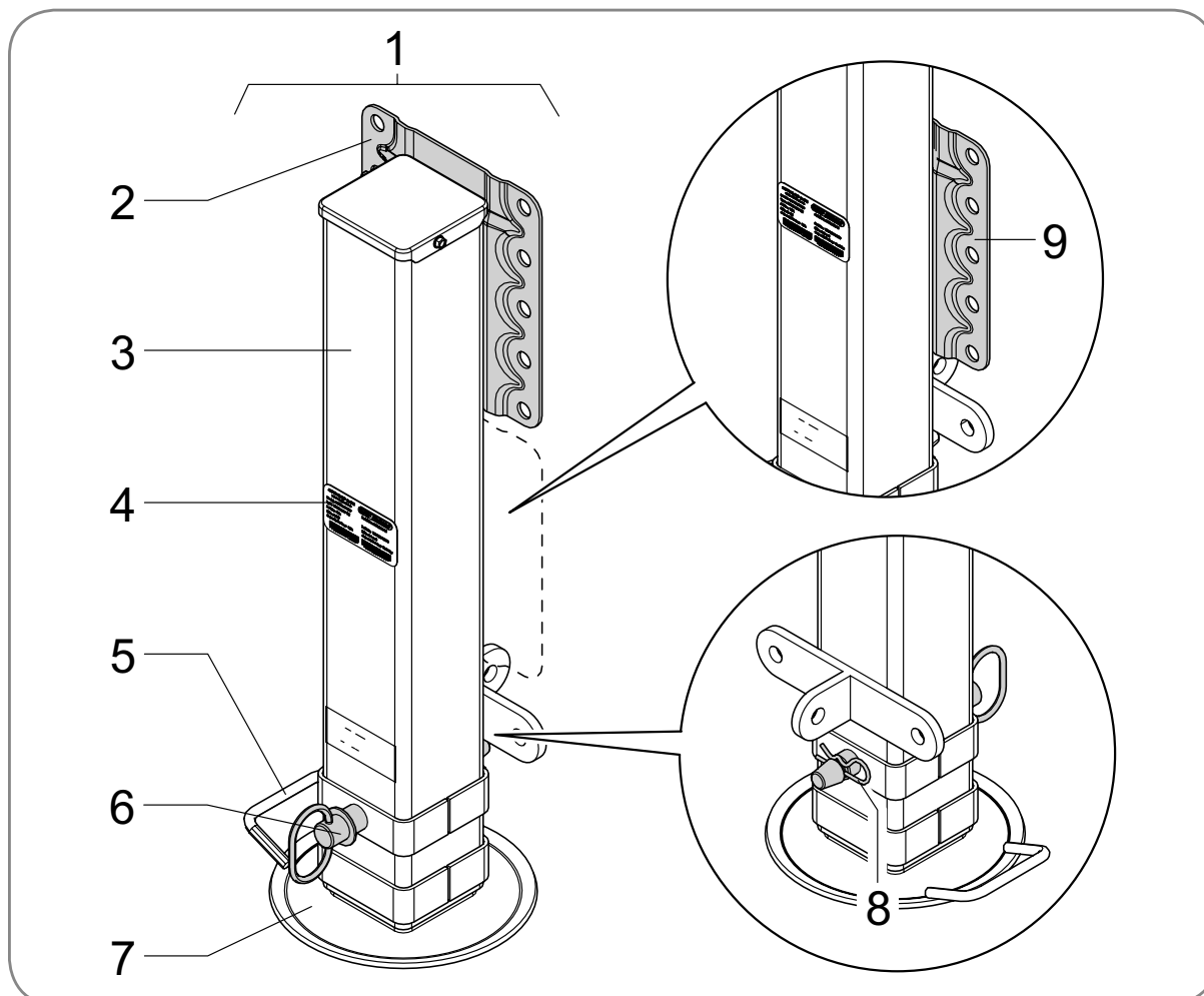
Abb. 3 - Bauteilübersicht SAF Fallstütze
