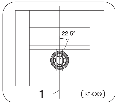
Abb. 8 · Einbauvorschlag für Zugsattelzapfen
