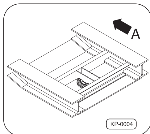
Abb. 9 · Beispiel für Einbaulage in Fahrtrichtung
