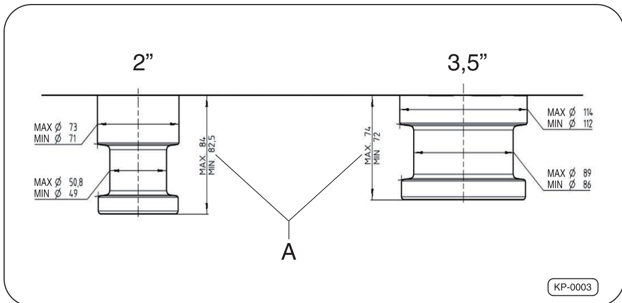
Abb. 11 · Verschleißkontrolle Zapfen
