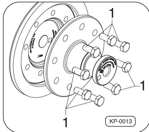
Abb. 12 · Anzugsdrehmoment Zugsattelzapfen
