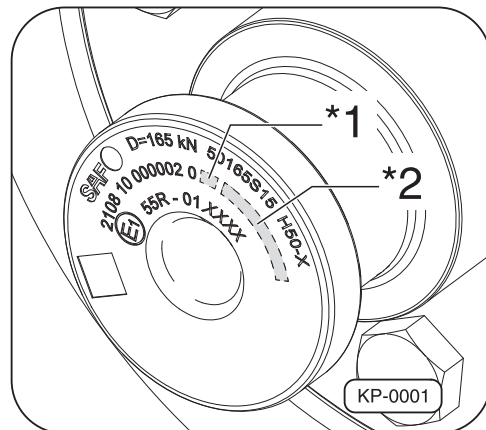
Abb. 1 · Zapfen Beispiel 50S15
