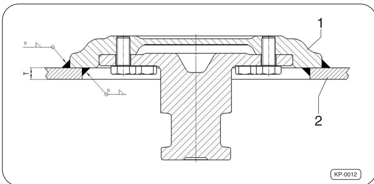
Abb. 6 · Flansch verschweißen
