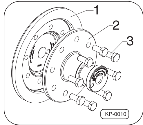
Abb. 7 · Montageübersicht Zugsattelzapfen
