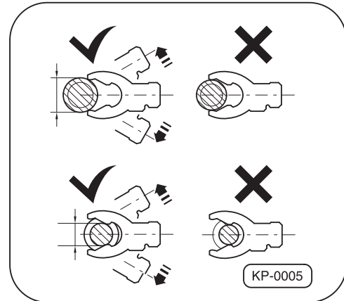
Abb. 10 · Verschleißkontrolle Grenzmaßlehre
