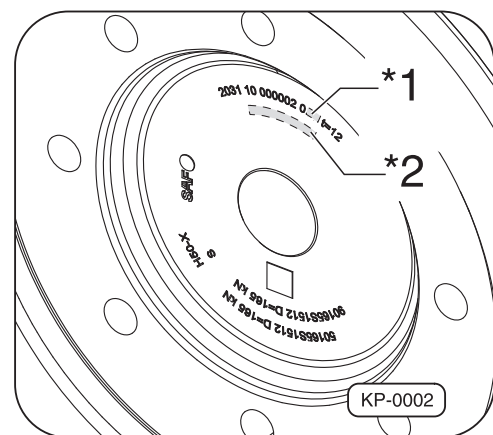
Abb. 2 · Flansch Beispiel 50S15 bzw. 90S15
